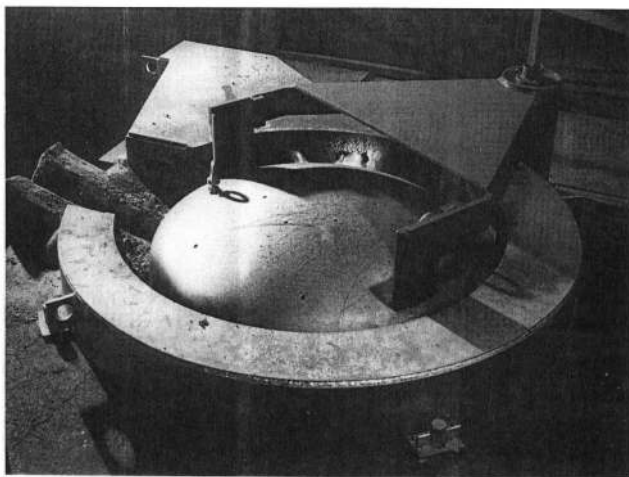
Bild 7: MF-Ind.-Tiegelofen mit Tiegelrandabsaugung
