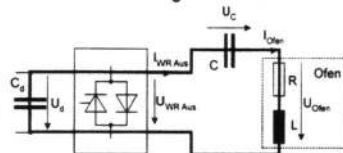
Reihenschwingkreisumrichter
