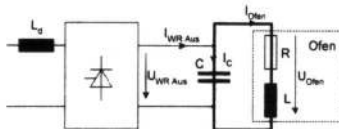
Parallelschwingkreisumrichter
