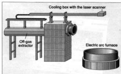
Fig. 2. Schematic diagram of the LaCam manipulator unit Bild 2. Schematische Darstellung des Laser-Manipulators
