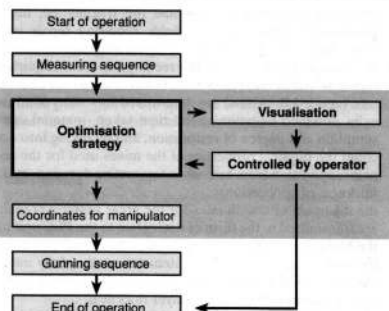
Fig. 4. Scantrol process (schematic) Bild 4. Der Scantrol-Prozess
