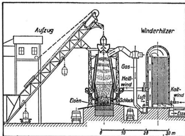
Bild 1. Schematische Darstellung einer Hochofenanlage Blast furnace
