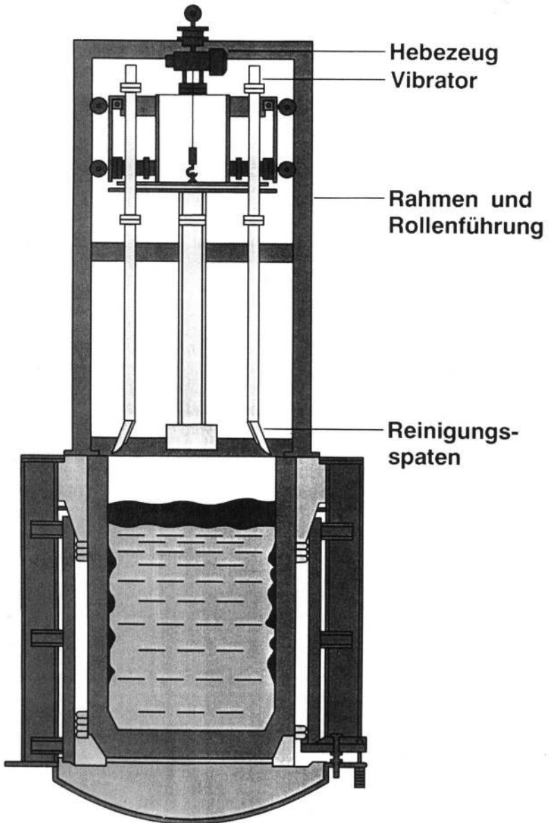
Tiegelreinigungsgerät
